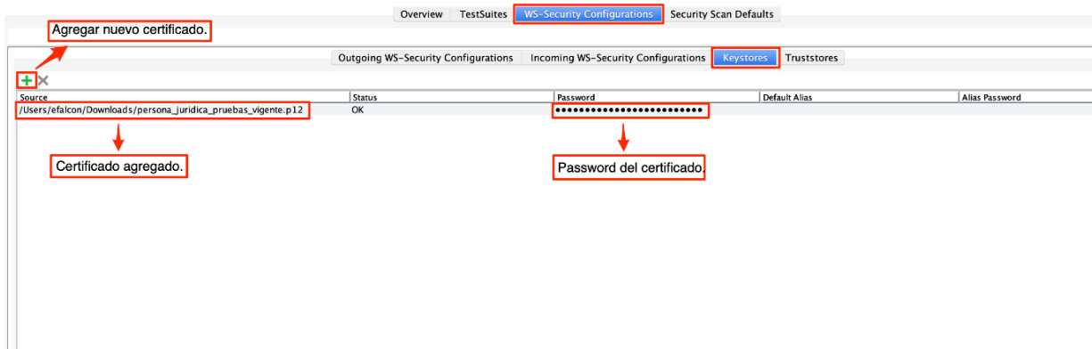
Ilustración 4. Configuración keystore
